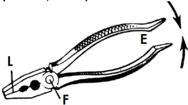
b) Pliers / Pair of pliers
